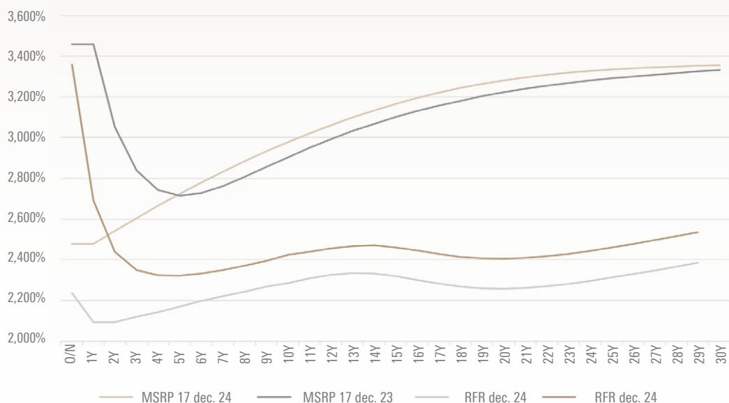
Slika 3: Netvegana krivulja RFR, diskontna krivulja MSRP 17 in premija za nelikvidnost na 31. 12. 2024 in 31. 12. 2023
